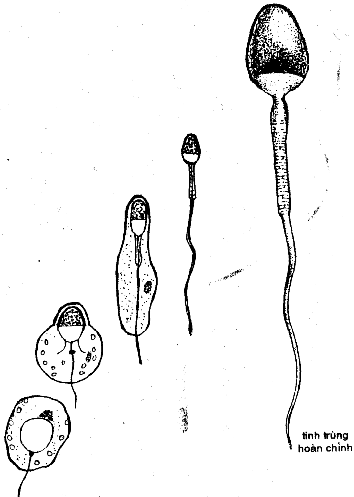
Hình 12 : Sinh tinh
