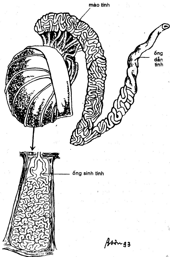
Hình 10 : Tinh hoàn
